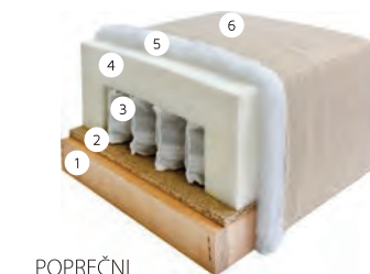
POPREČNI PRESEK SEDIŠTA
